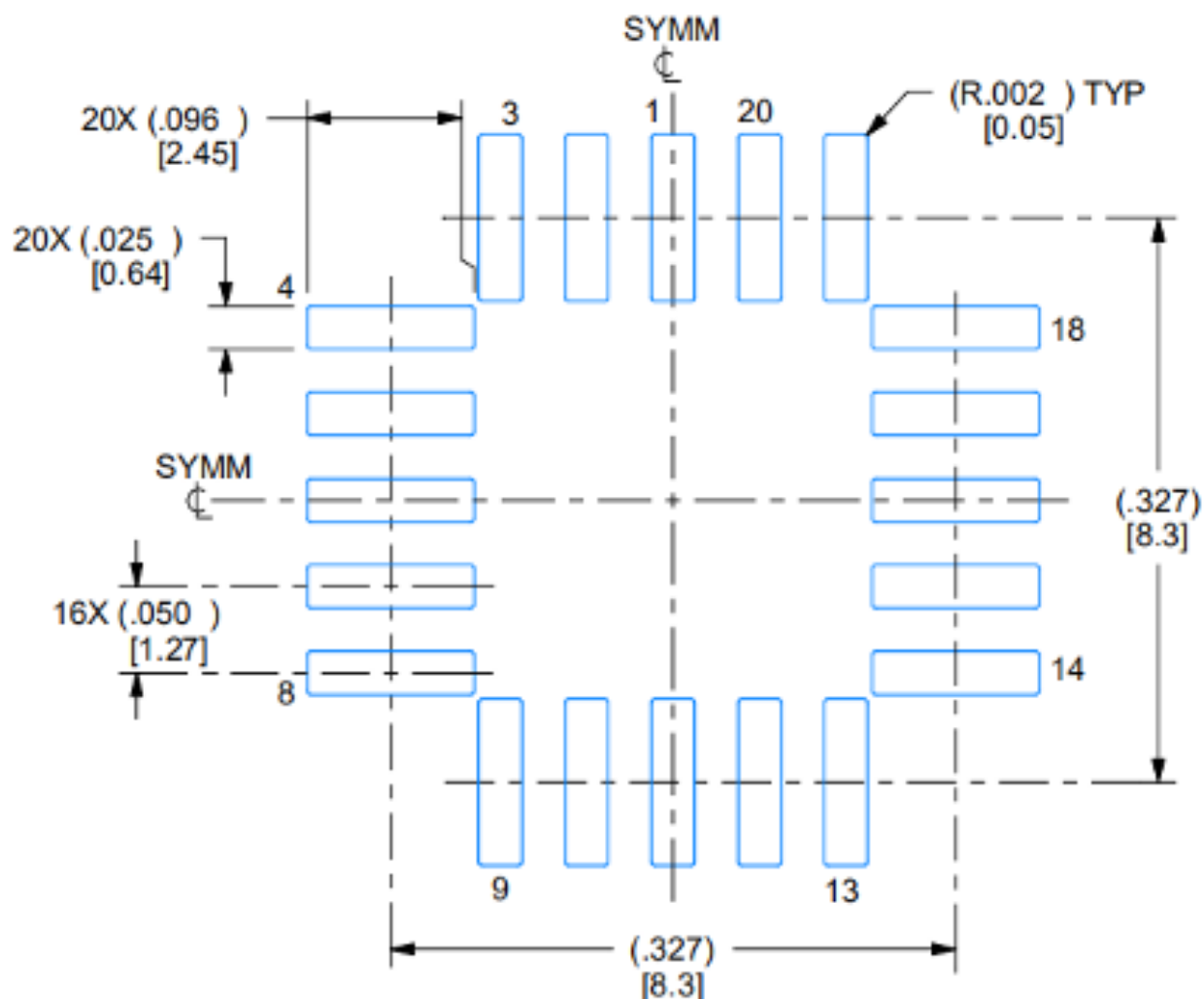
焊盘布局示例 尺寸：6倍
