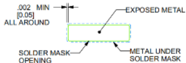
定义的焊接面
