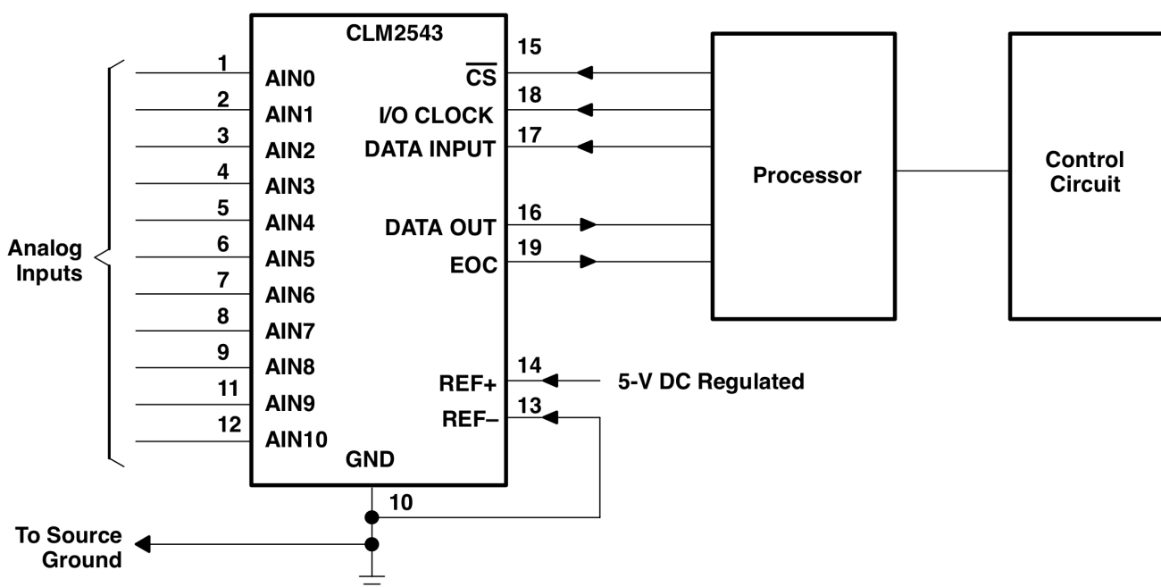
图17.串行接口
