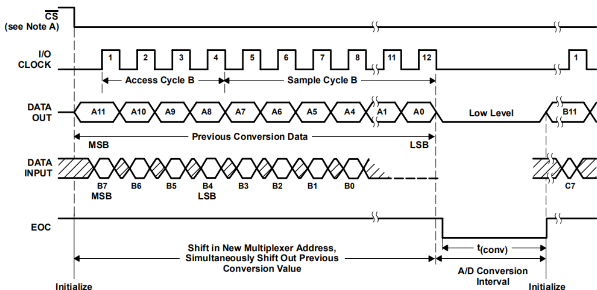
图9.首先使用和MSB进行12时钟传输的时序
