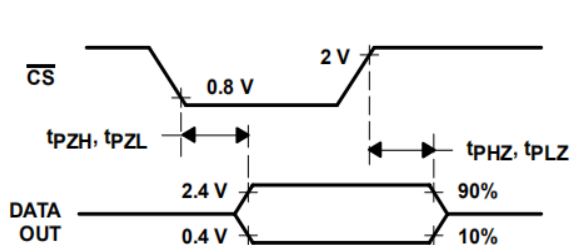
图3.数据输出到Hi-Z电压波形
