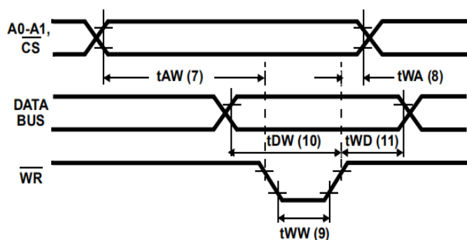
图30.写时序
