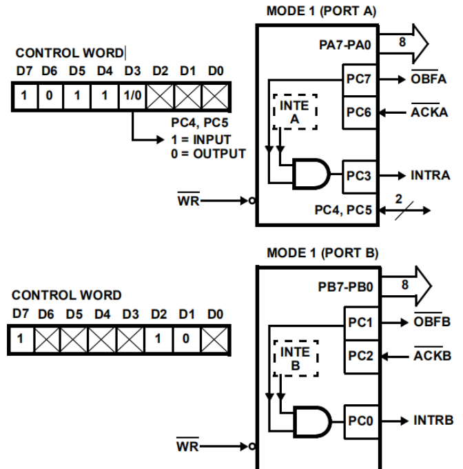
图8. 模式1输出
