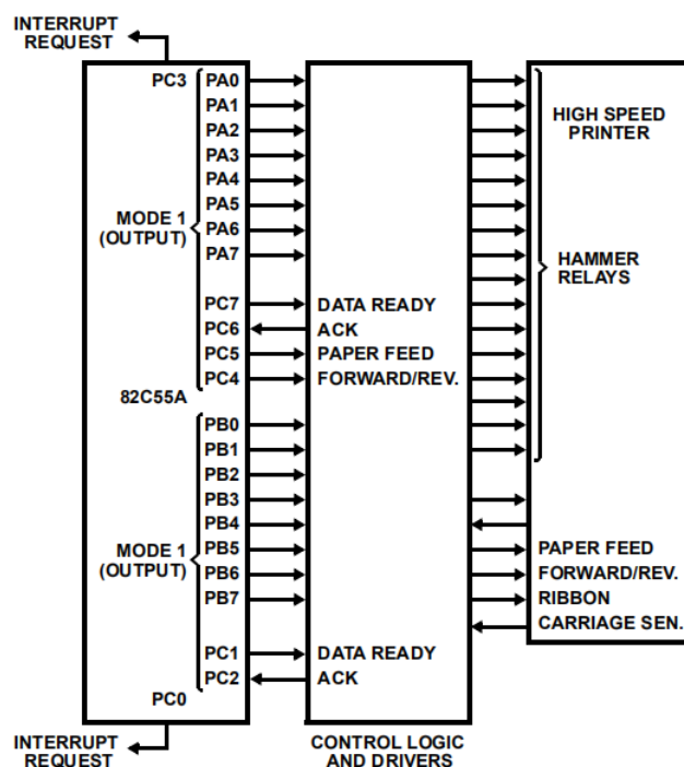
图18.打印机接口
