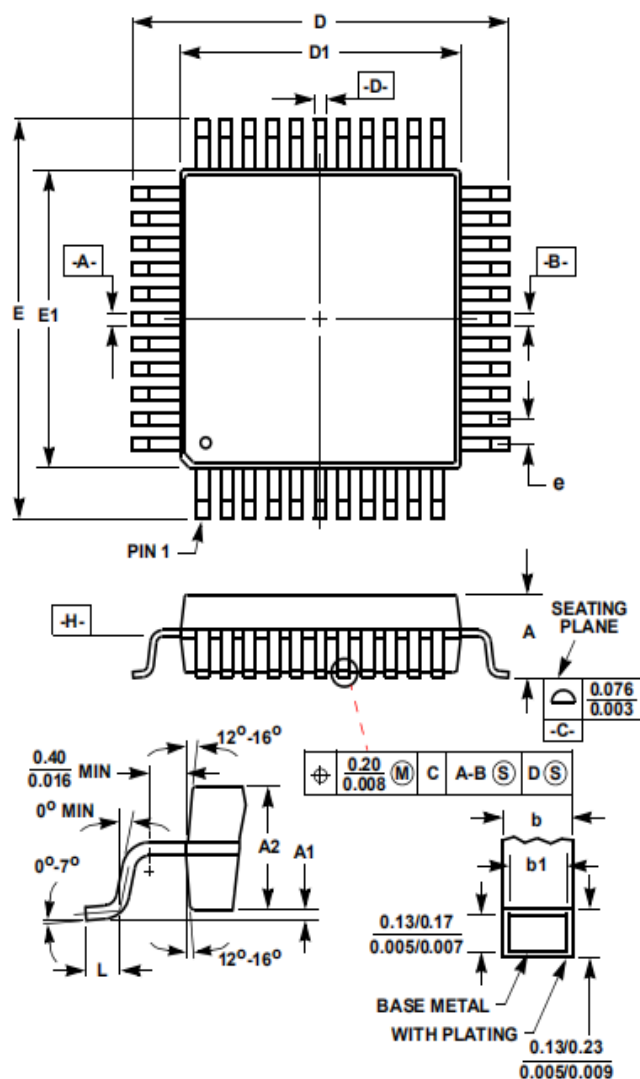
Q44.10x10 ( JEDEC MS-022AB问题B ) 44铅公制塑料四边行背包包装
