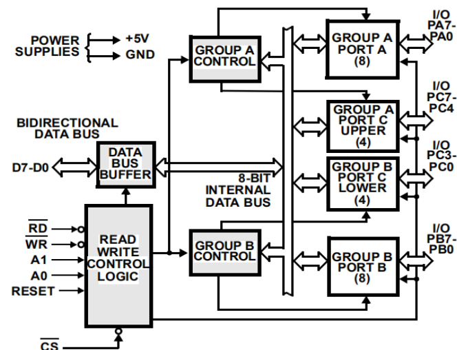
图1. 82C55A框图。数据总线缓冲，读/写，A组和B组控制逻辑功能
