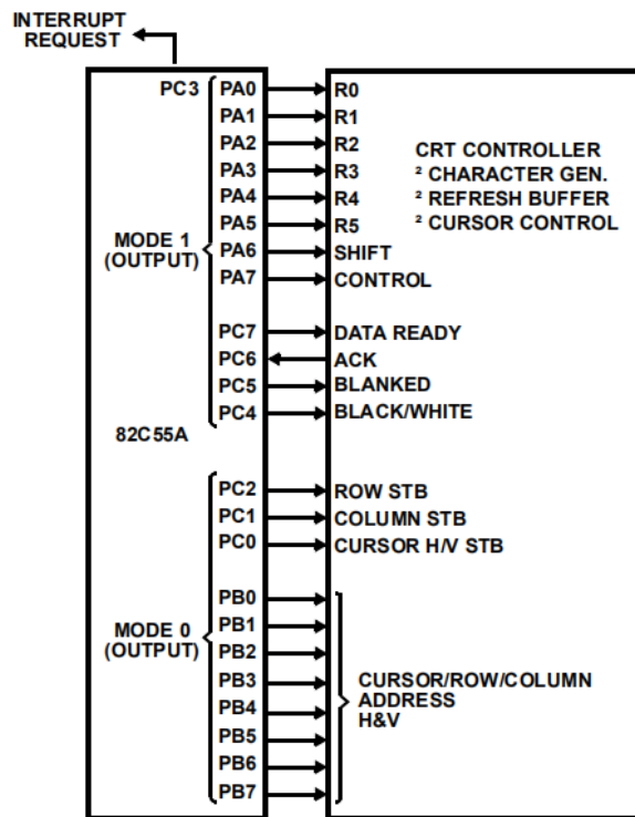
图22. 基本的CRT控制器接口
