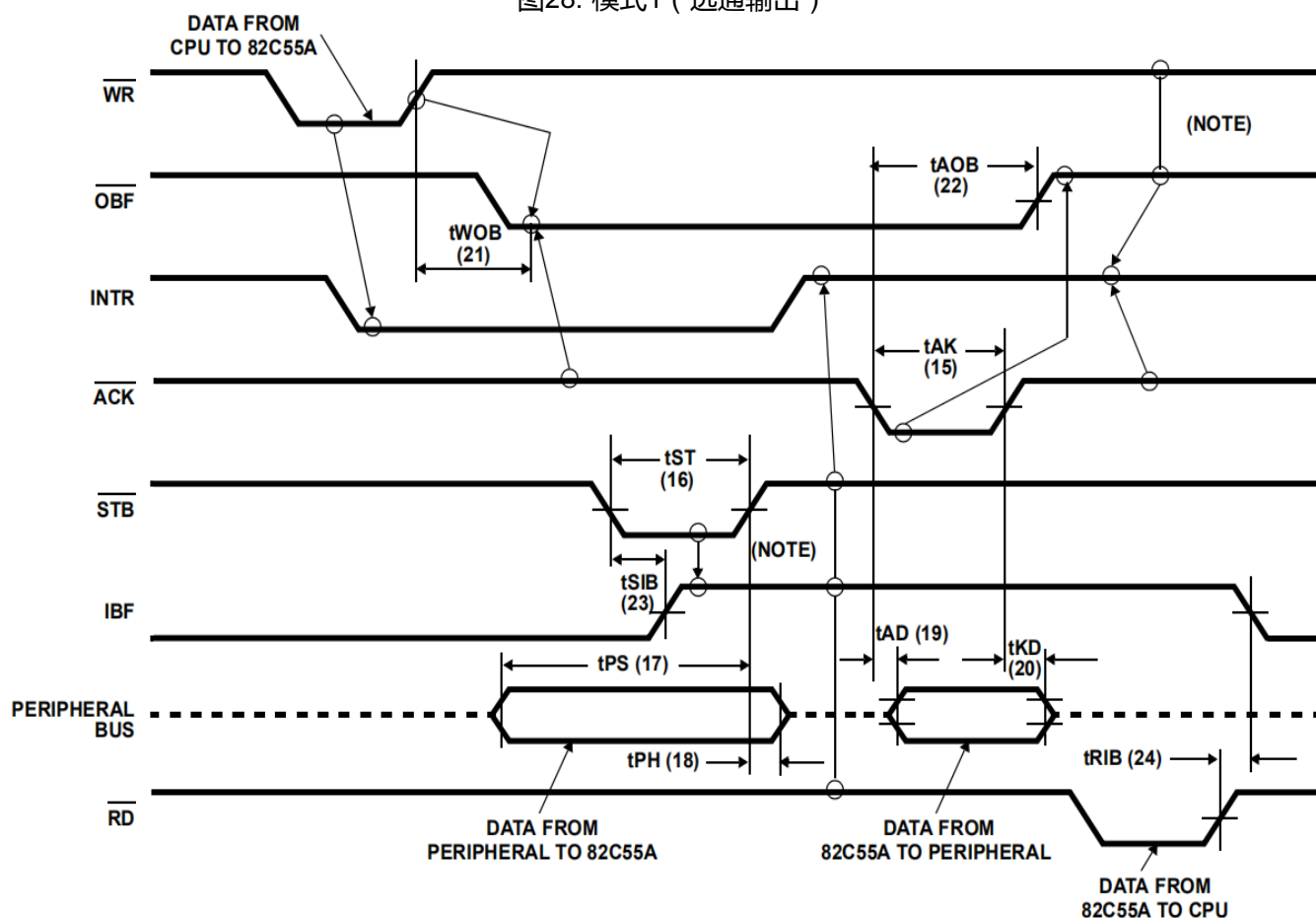
图29. 模式2 ( 双向 )
