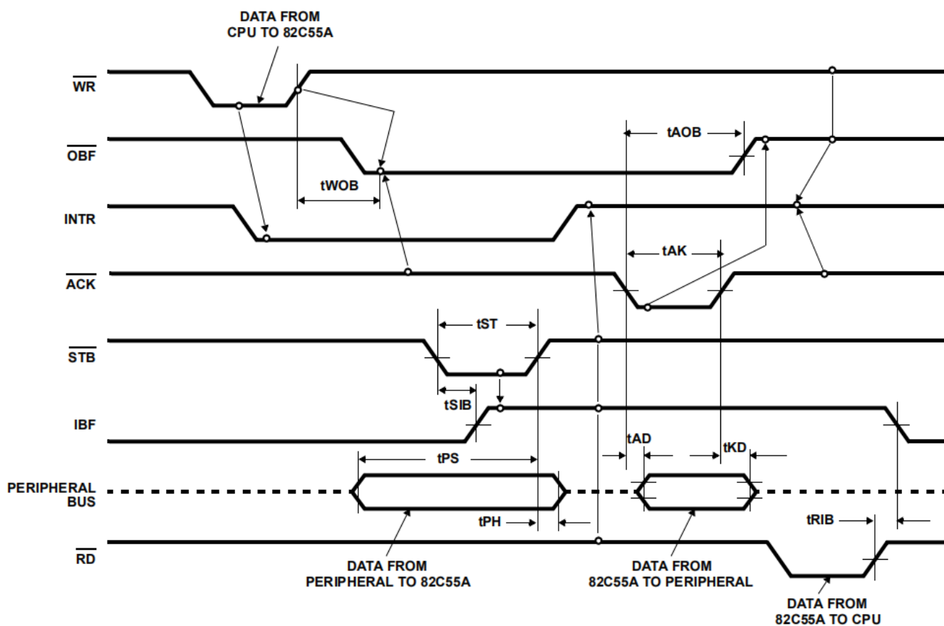
图13. 模式2 (双向)
