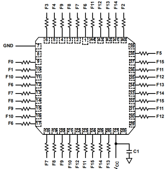
CLCC
