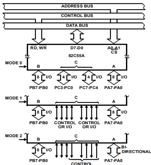
图3. 基本模式定义和总线接口
