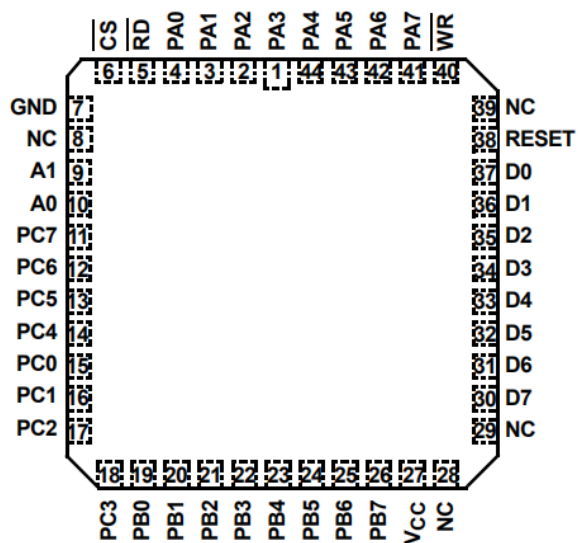
82C55A(CLC) 顶视图
