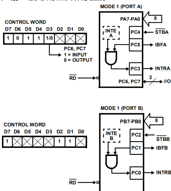
图6. 模式1输入
