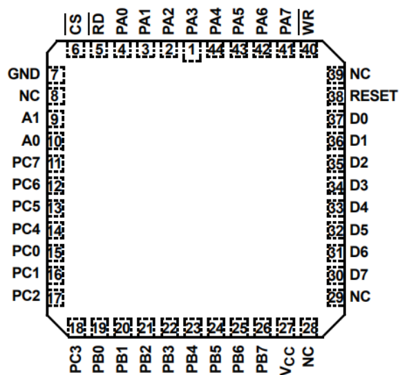
82C55A(CLCC) 顶视图
