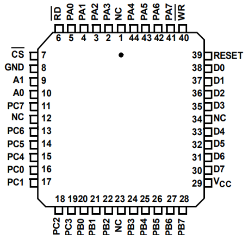
82C55A(PLCC) 顶视图
