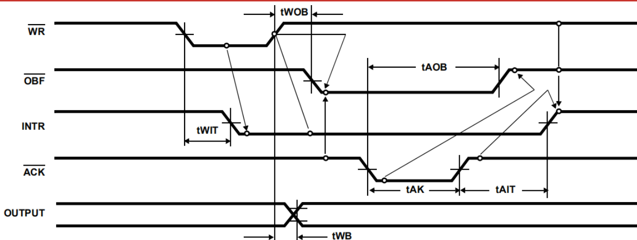
图9. 模式1 ( 选通输出 )
