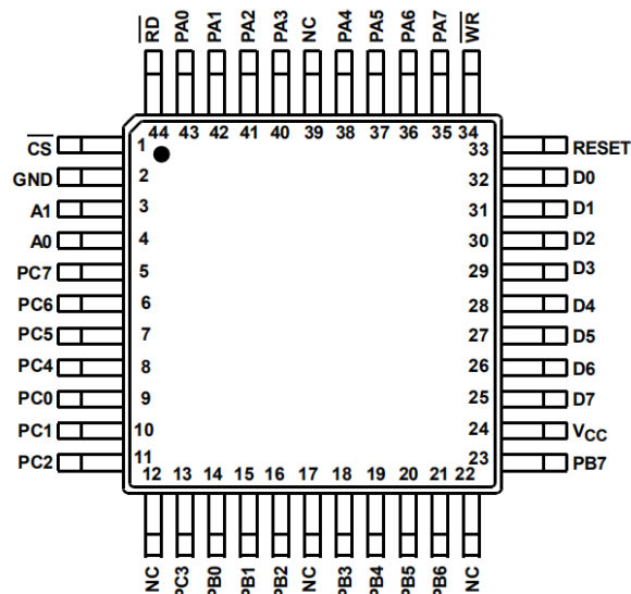
82C55A(MQFP) 顶视图
