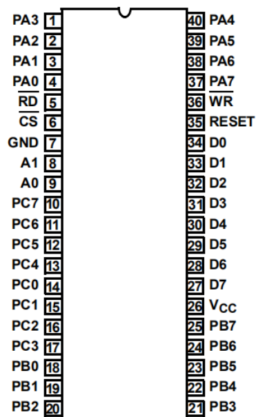
82C55A(PDIP,CERDIP) 顶视图
