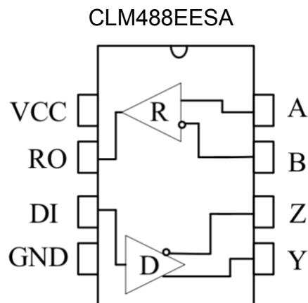
图 1 CLM488EESA 引脚分布图
