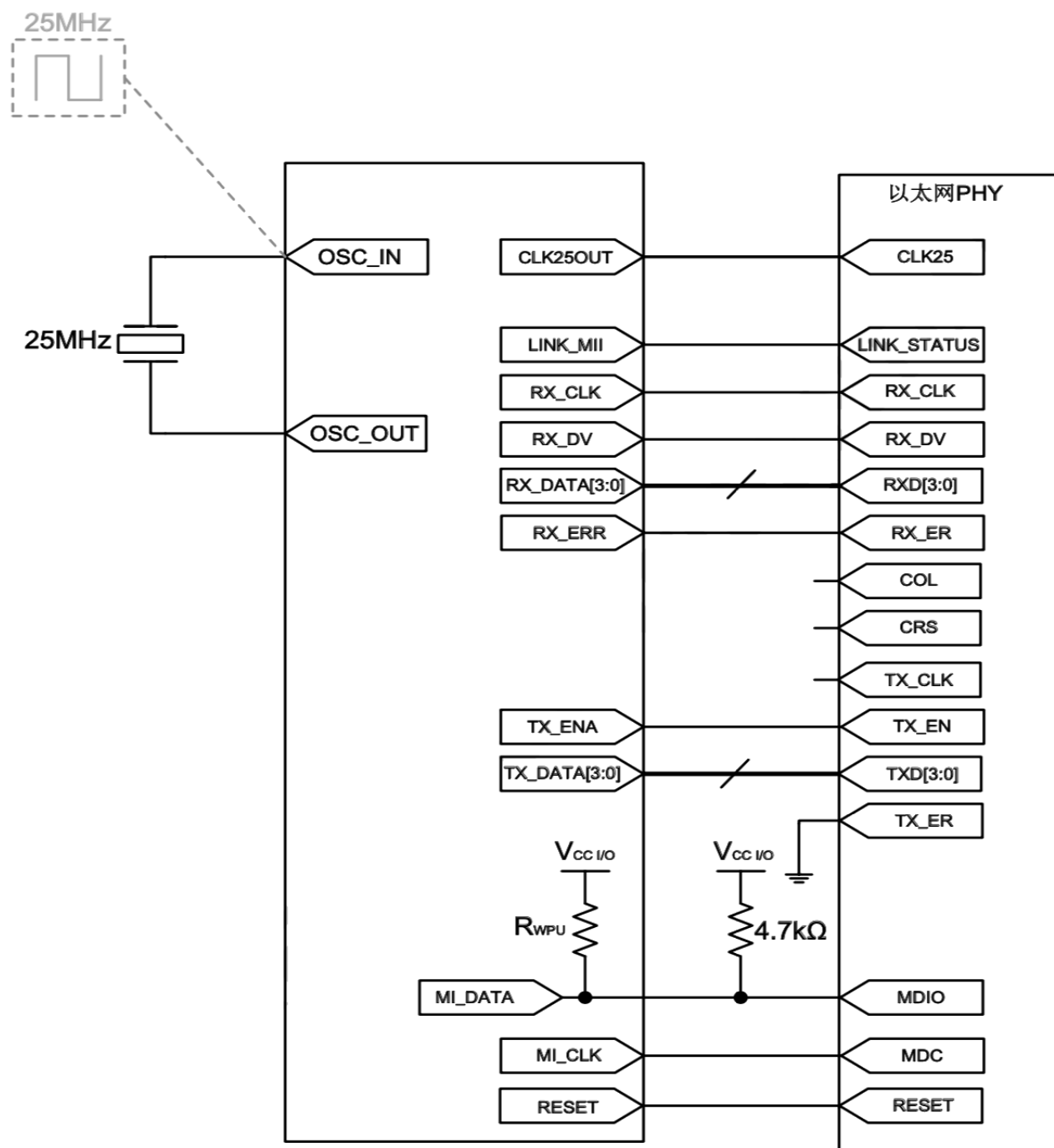
图 3-10 PHY 连接
