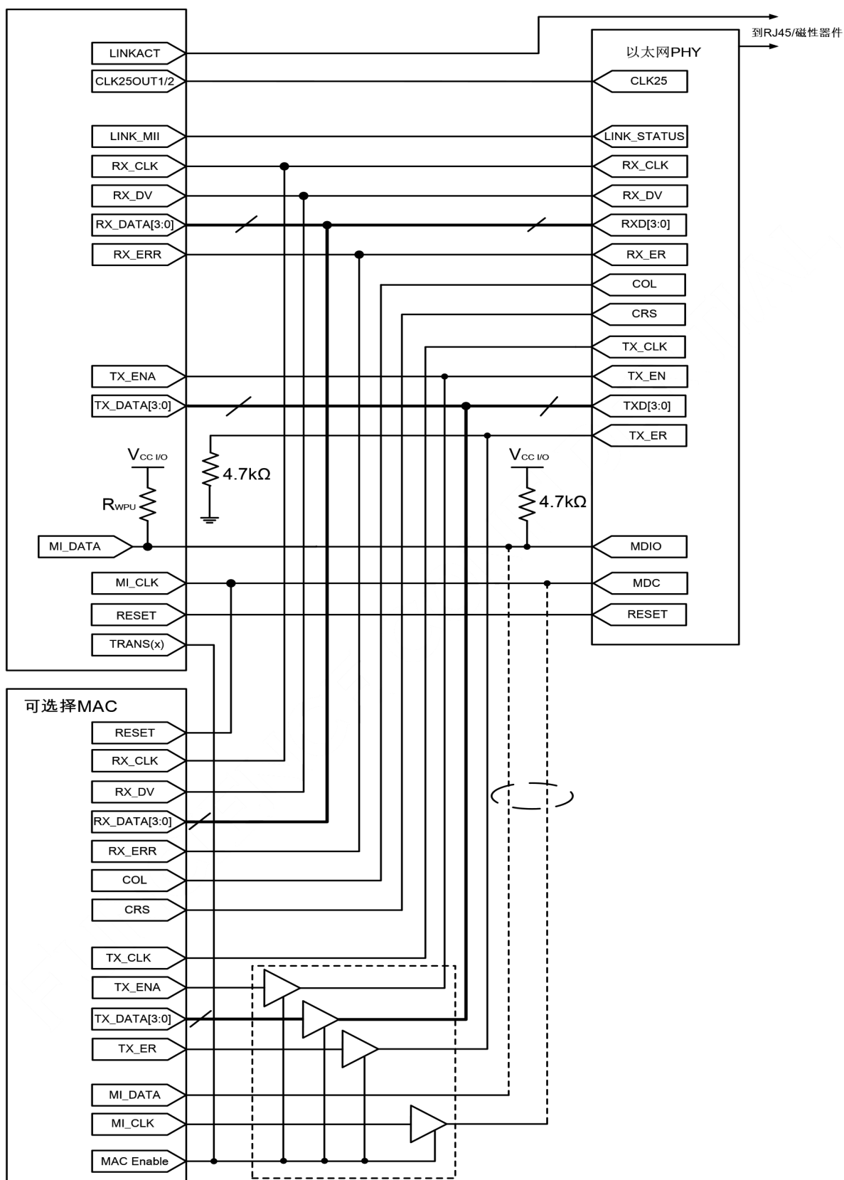
图 3-9 透明模式
