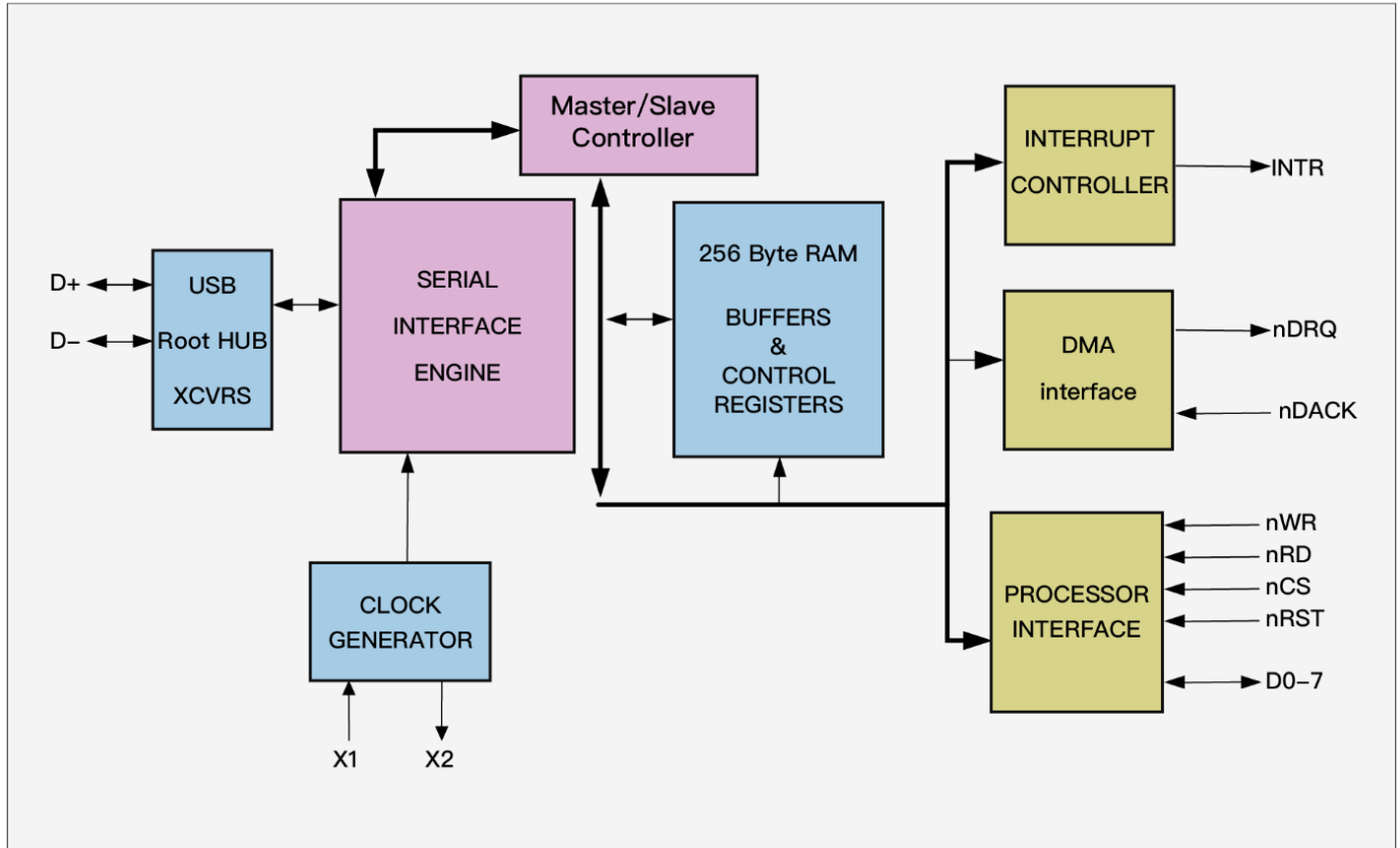
CLM811HST-AXC框图
