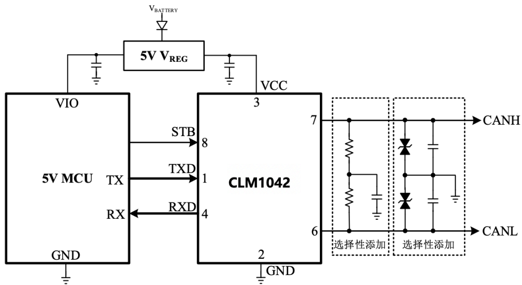
图 6 CLM1042AT 与 5V MCU 典型应用图
