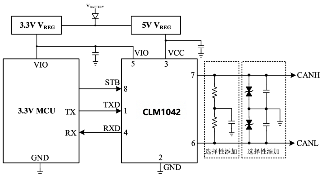
图 7 CLM1042AT/3 与 3.3V MCU 典型应用图
