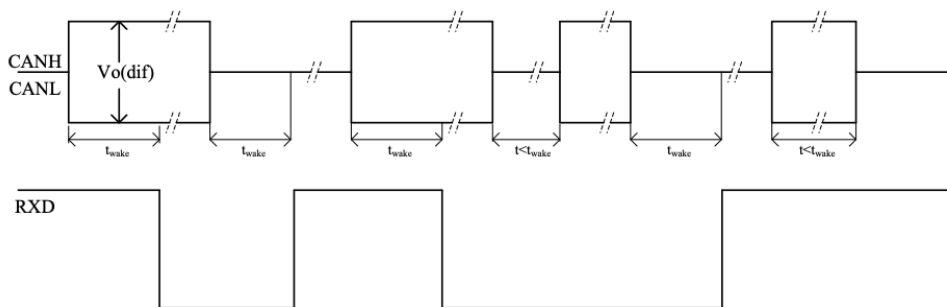
图 8 唤醒时序
