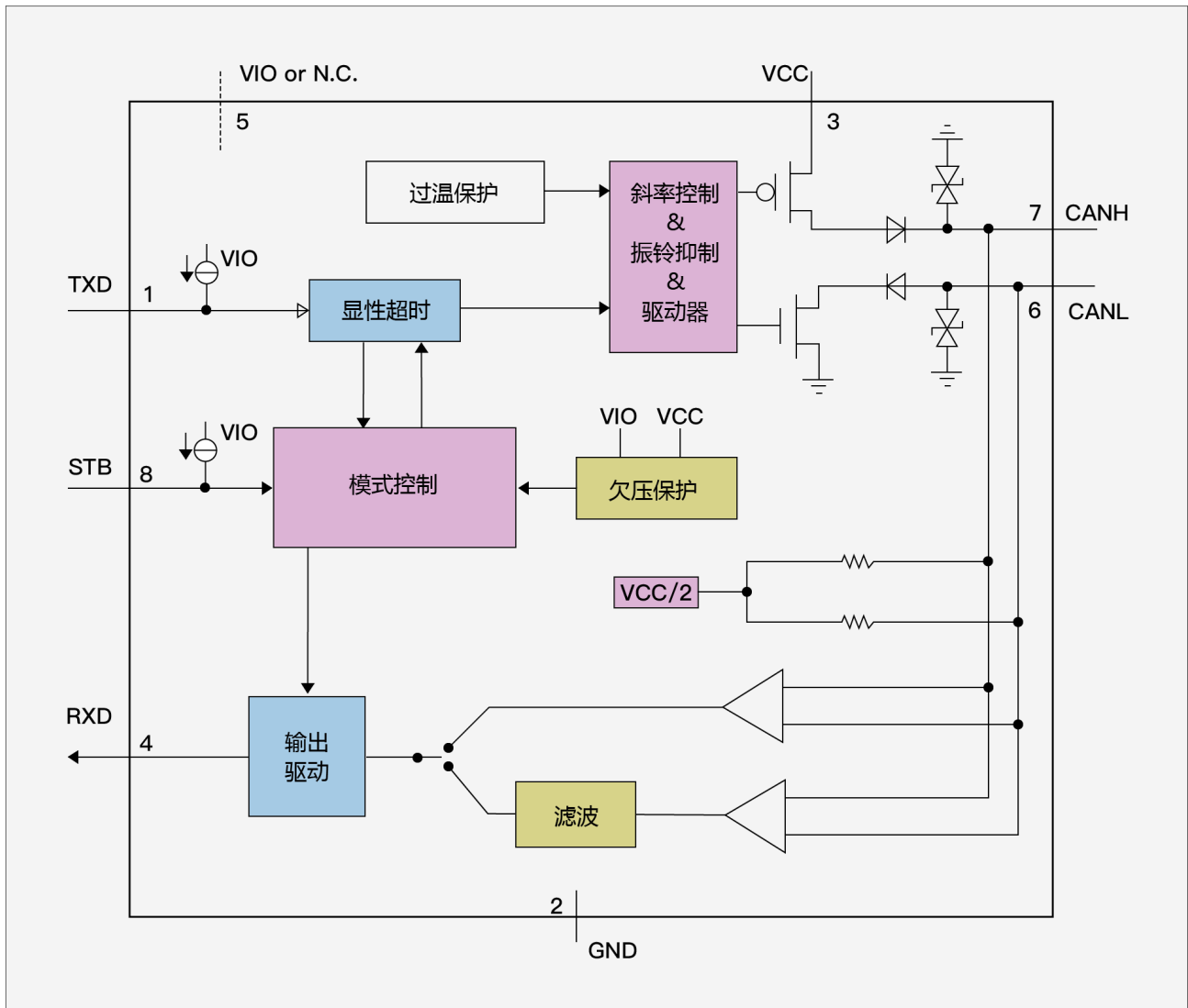
CLM1042框图
