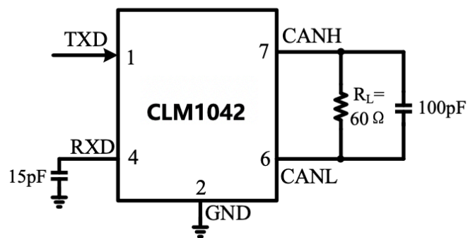
图 4 收发器时序测试电路图
