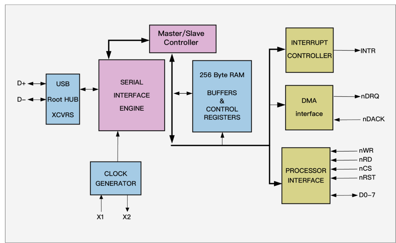
CLM811HST-AXC框图
